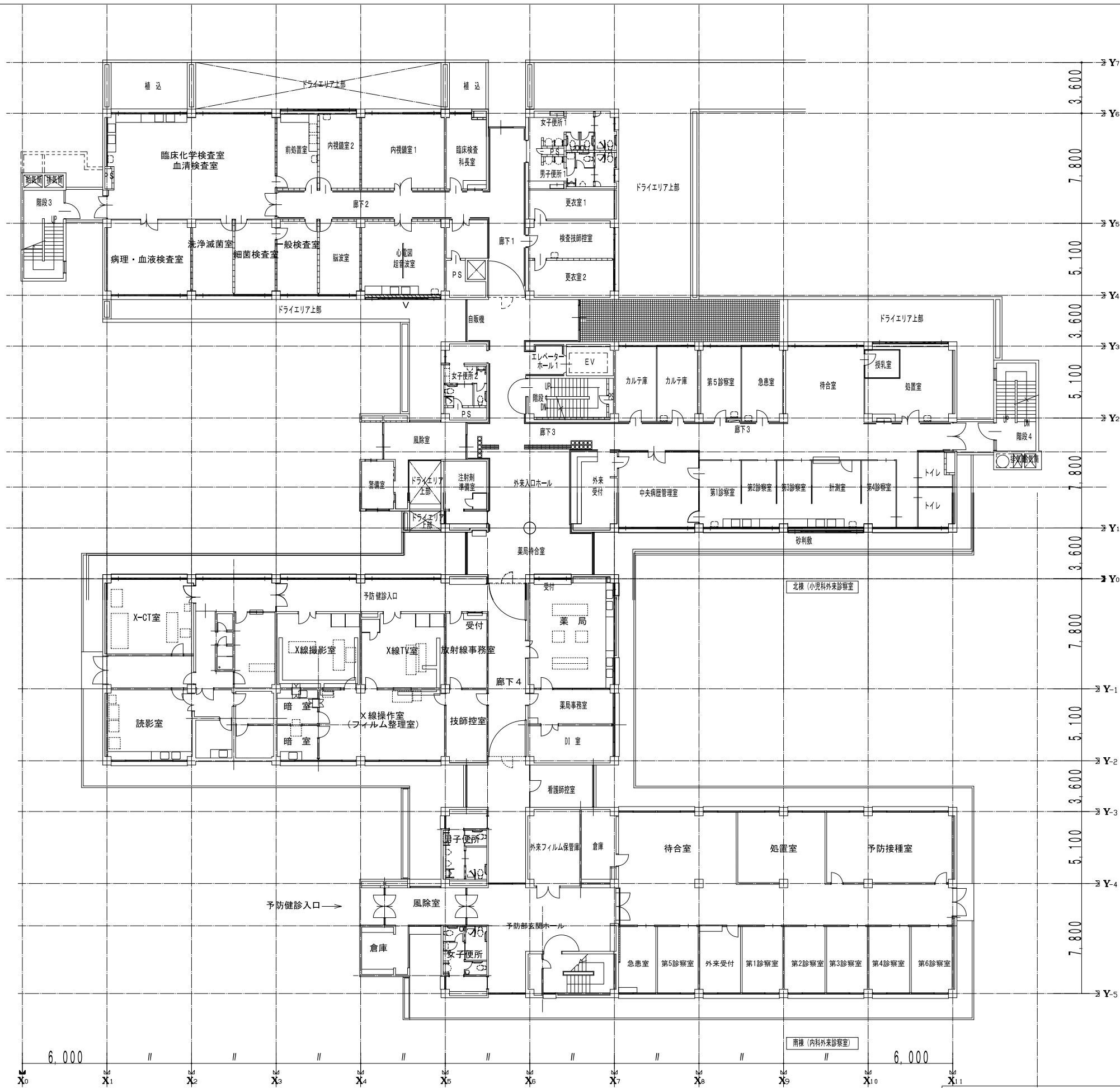
北棟 1階平面図
